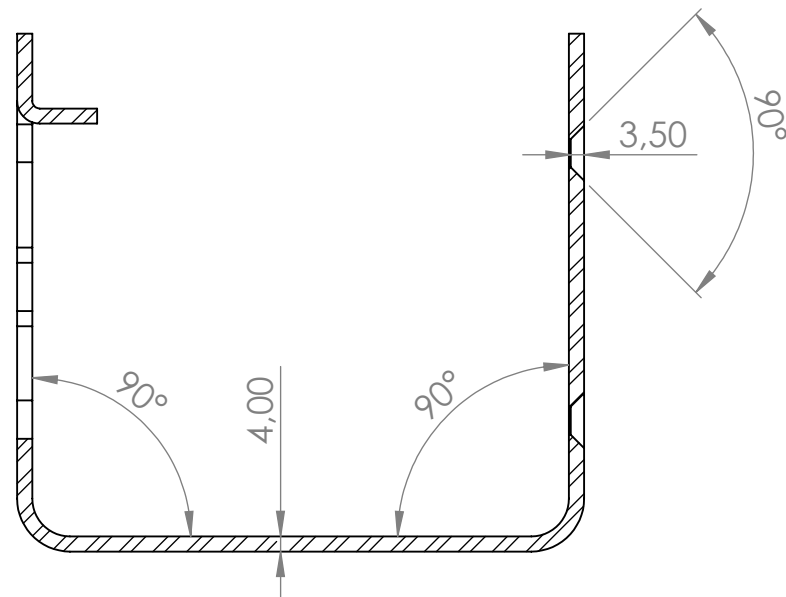
COUPE D-D
